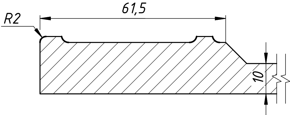
Сечение профиля
