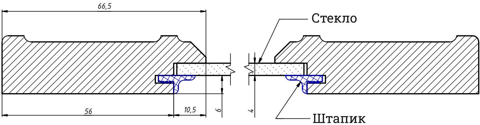
Сечение профиля
