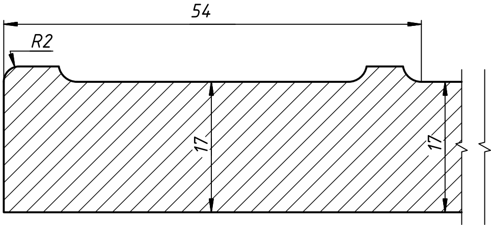
Сечение профиля
