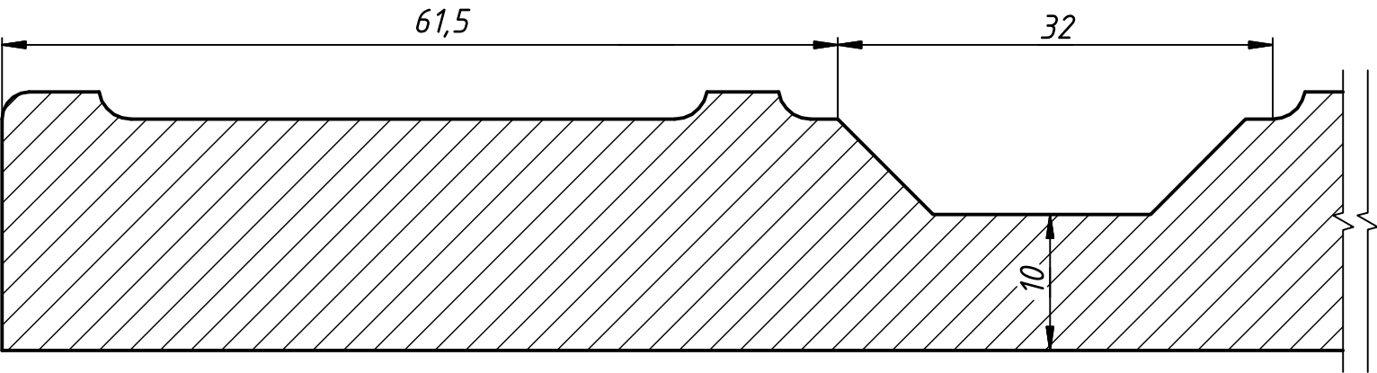
Сечение профиля
