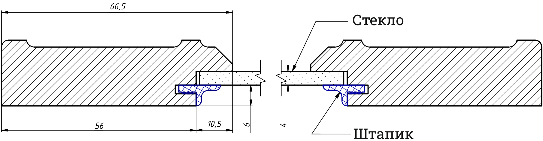
Сечение профиля
