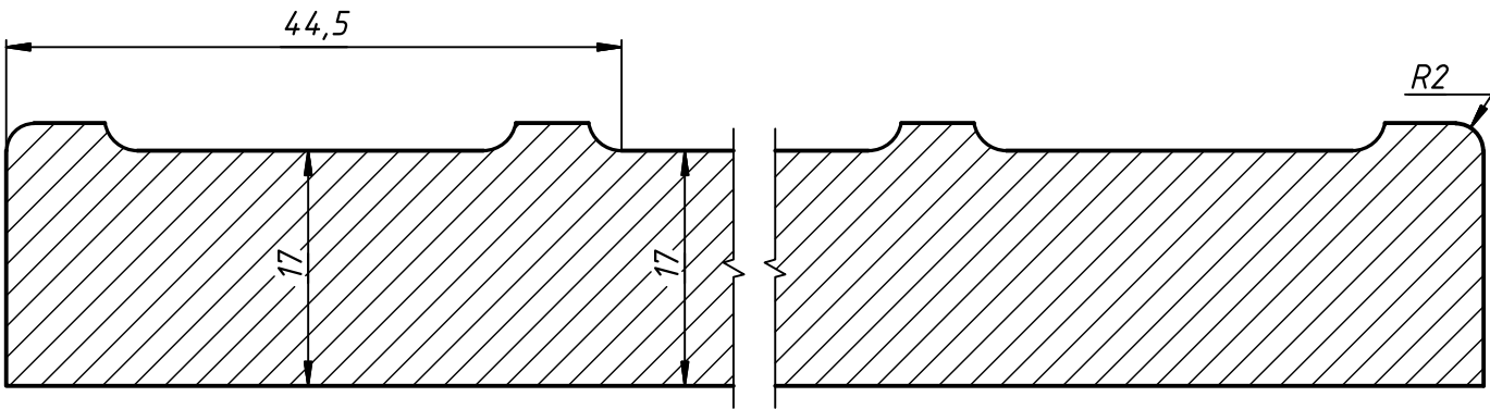
Сечение профиля
