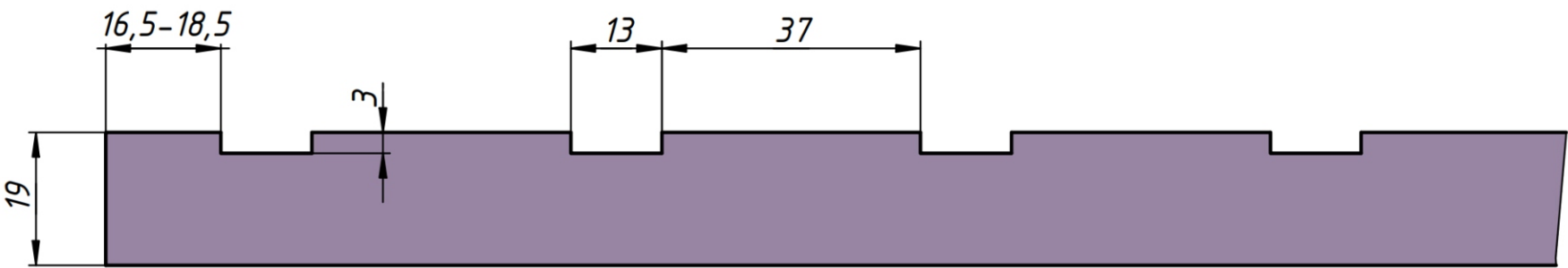
Сечение профиля. Шаг повторения фрезы 50мм.
