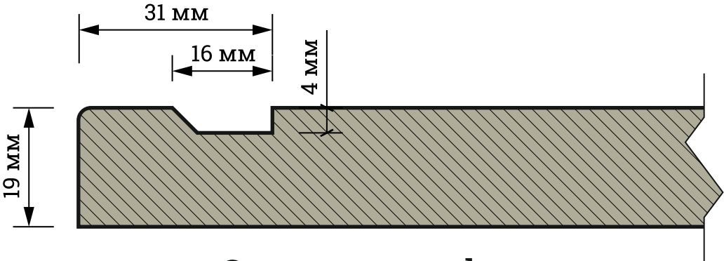
Сечение профиля
