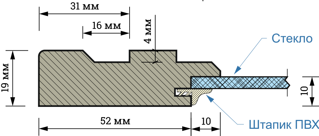
Сечение профиля
