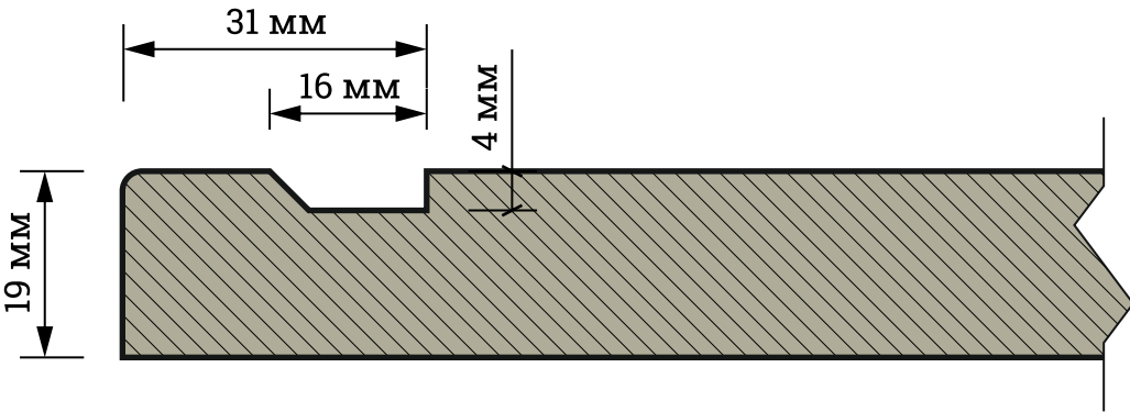
Сечение профиля
