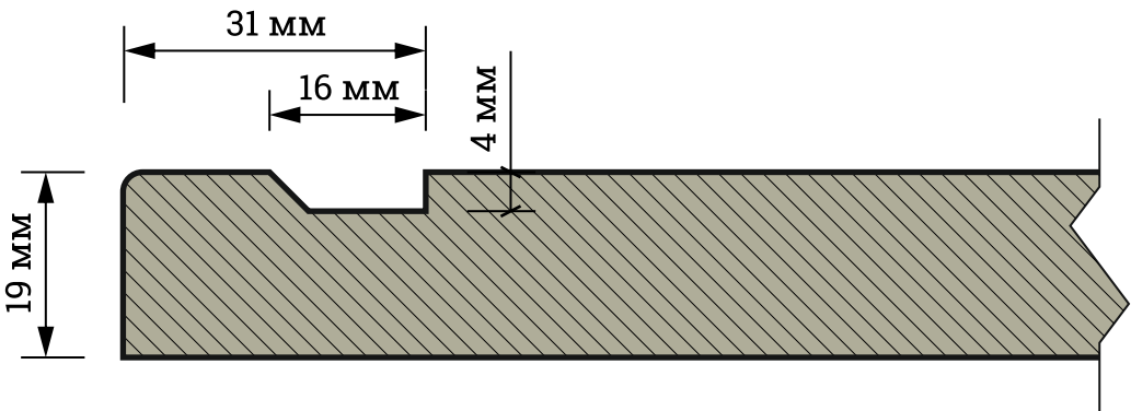
Сечение профиля
